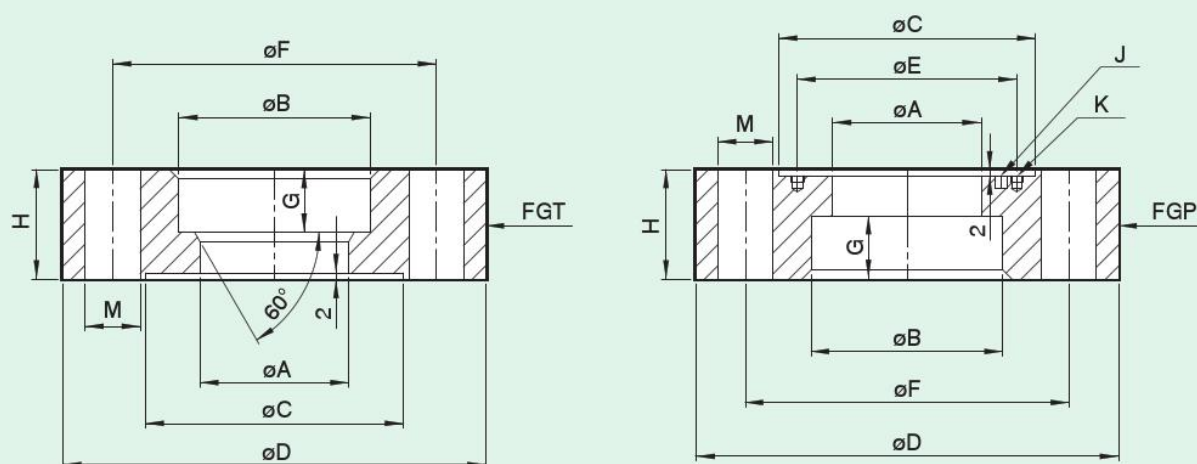
Flanges Dimensions (mm) 碟式預充閥安裝法蘭參考尺寸
